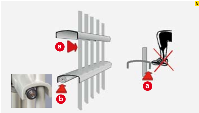
5. adronit®-Sicherheitszaun IntelliFence®, eine gelungene Kombination aus mechanischem Schutz und elektronischer Detektion: a. Außermittig angebrachte Rundstäbe machen das U-Profil asymmetrisch und erschweren ein Übersteigen stark b. Verdeckte Unterbringung des Detektionskabels im U-Profil
