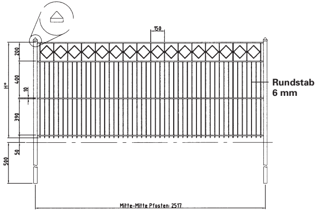
Schmuckzaun ARTE STELLA-SL
