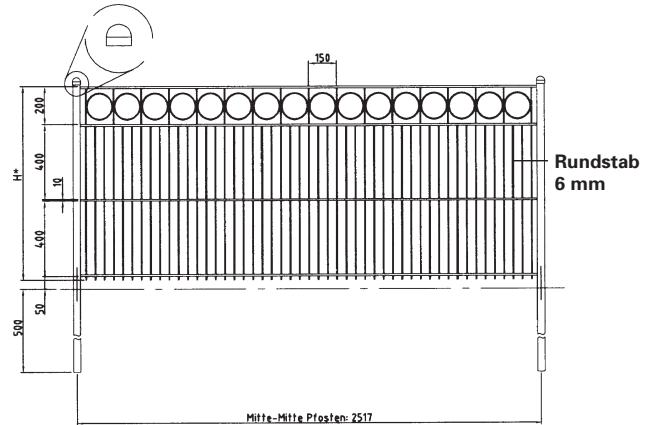
Schmuckzaun ARTE STELLA-SL
